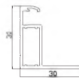
Схема розрізу довгого профілю рами
